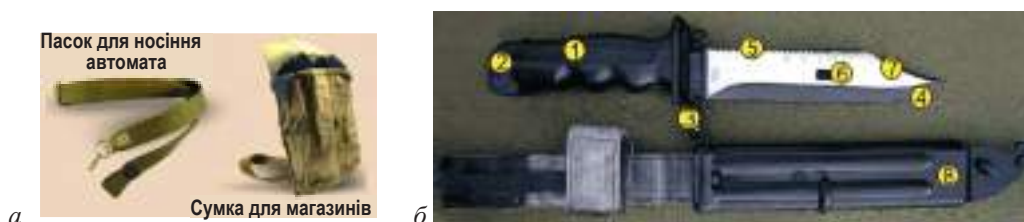
Лл. 18.4. Комплект для автомата Калашнікова: а — сумка для магазинів, пасок для носіння автомата; б — багнет-ніж: 1 — ручка; 2 — кнопка фіксатора; 3 — кільце; 4 — лезо; 5 — шпилька; 6 — отвір; 7 — ріжуча грань; 8 — піхва
