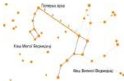
Іл. 31.5. Сузір'я Великої Ведмеді та Полярна зірка
