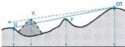
Лл. 33.9. Укриття нижче спостерігача (СП), але не вище цілі (Ц)
