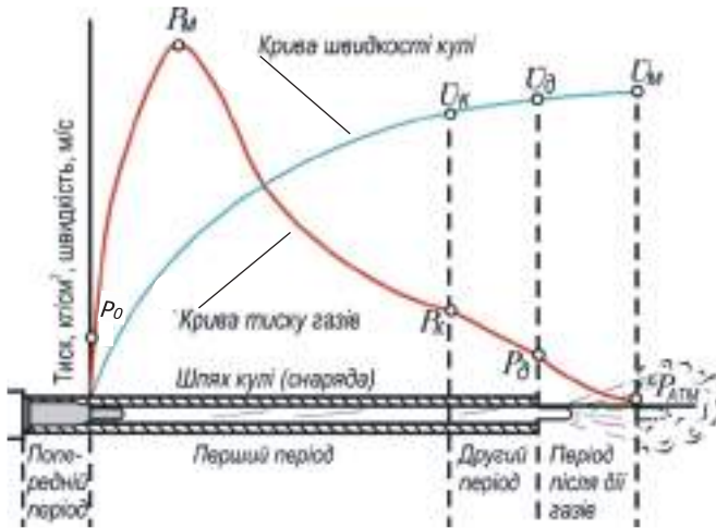
Іл. 16.1. Періоди пострілу
