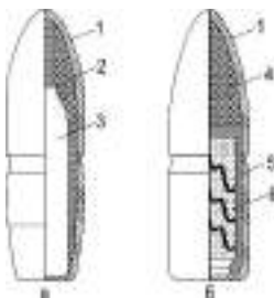
Іл. 22.4. Куля: а — звичайна зі сталевим осердям; б — трасуюча; 1 — оболонка; 2 — свинцева сорочка; 3 — сталеві серцевина; 4 — свинцева серцевина; 5 — стаканчик трасера; б — трасуюча суміш
